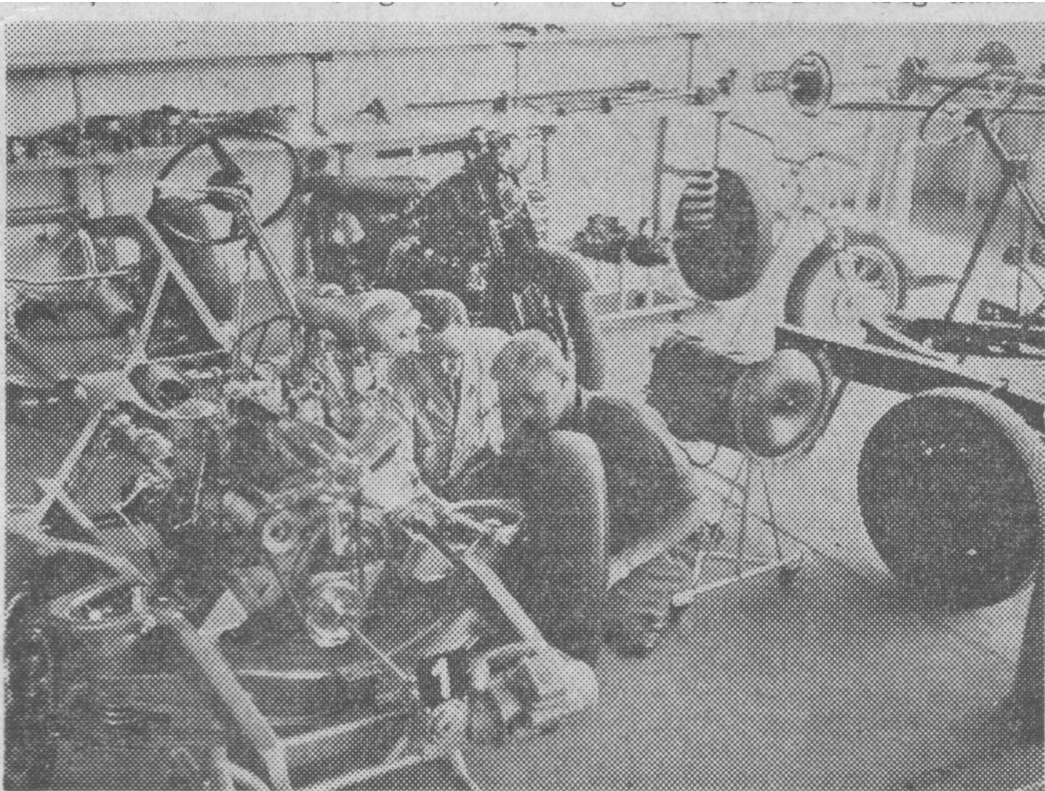
En udstrakt modelsamling er til raadighed for undervisningen og virker som overgangsled mellem praktik og teori. Her instruerer fænrik K. J. Sørensen i forhjulsaffjedring paa en Humber Hawk.
