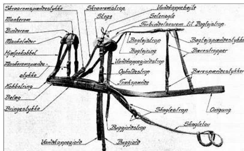
Trænsele M.1907.
