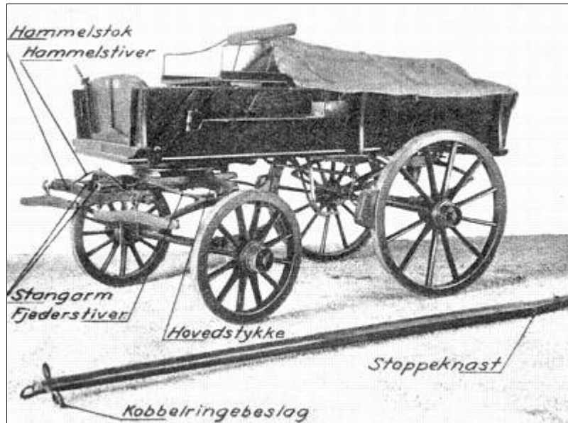
Trænvogn M.1909 2 ).
